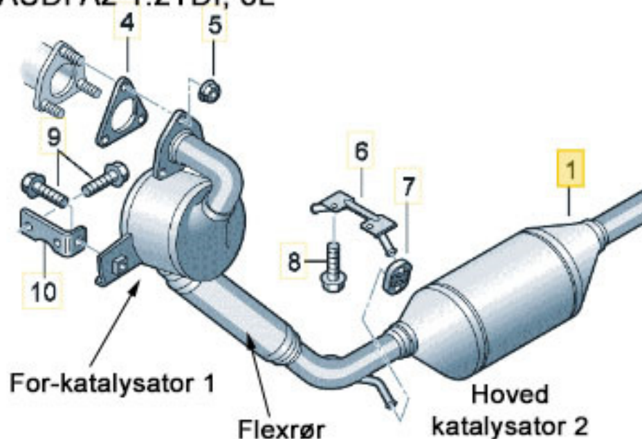
Original udstødning med 2 katalysatorer AUDI A2 1.2TDI, 3L
