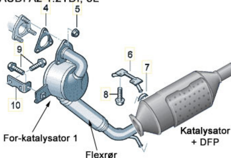
Udstødning med katalysator og DPF AUDI A2 1.2TDI, 3L
